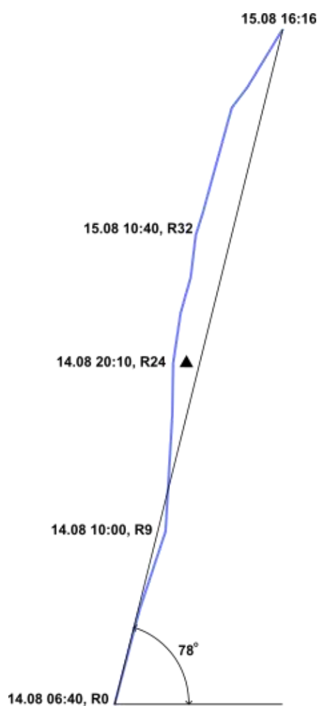
Рисунок 3: Рисованный профиль и техническая фотография маршрута. На участках R0-R32 использовалась одновременная схема движения со страховкой с перил. Все участки до R32 имеют длину не более 30 м.
